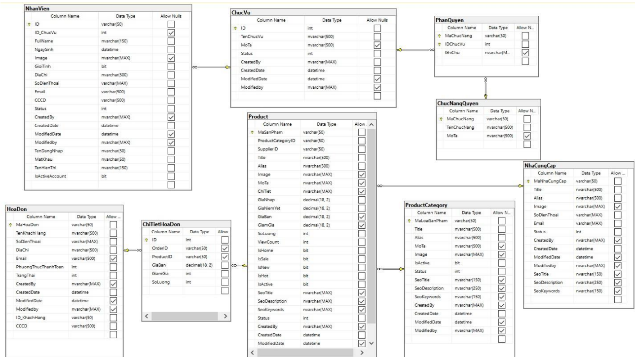
Hình 3.1. Sơ đồ logic được thiết kế bằng SQL Server
